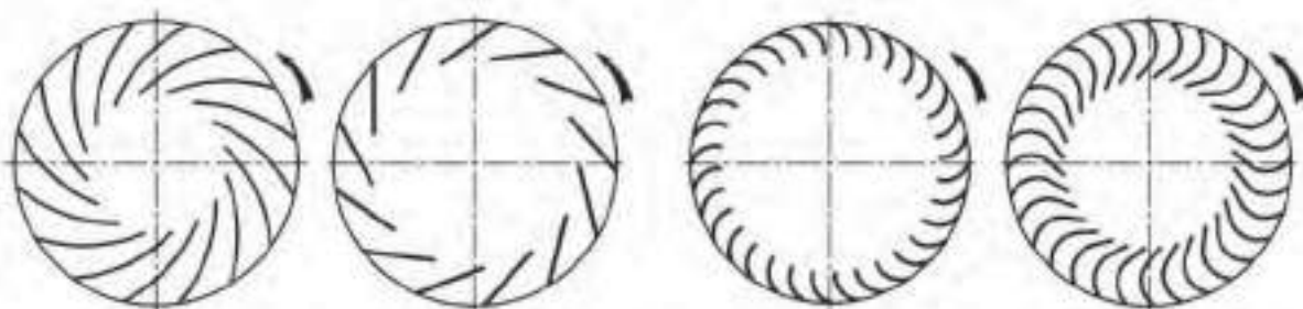
Назад загнутые лопасти
