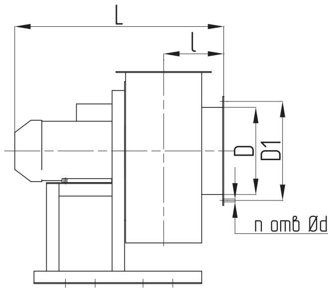
Схема расположения отверстий для крепления вентилятора ВЦП 7-40-2,5...3,15
