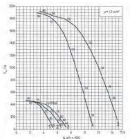
Аэродинамические характеристики ВКРФм ДУ; ДУВ 4,5
