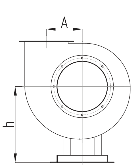
Выходной фланец
