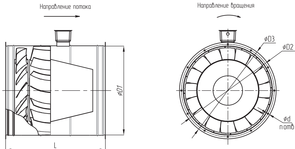
Компоновка 01
