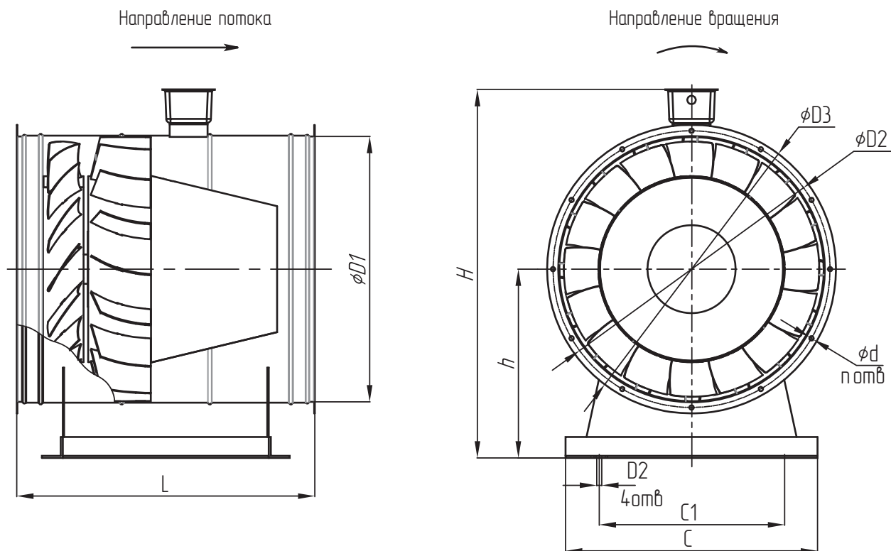
Компоновка 02
