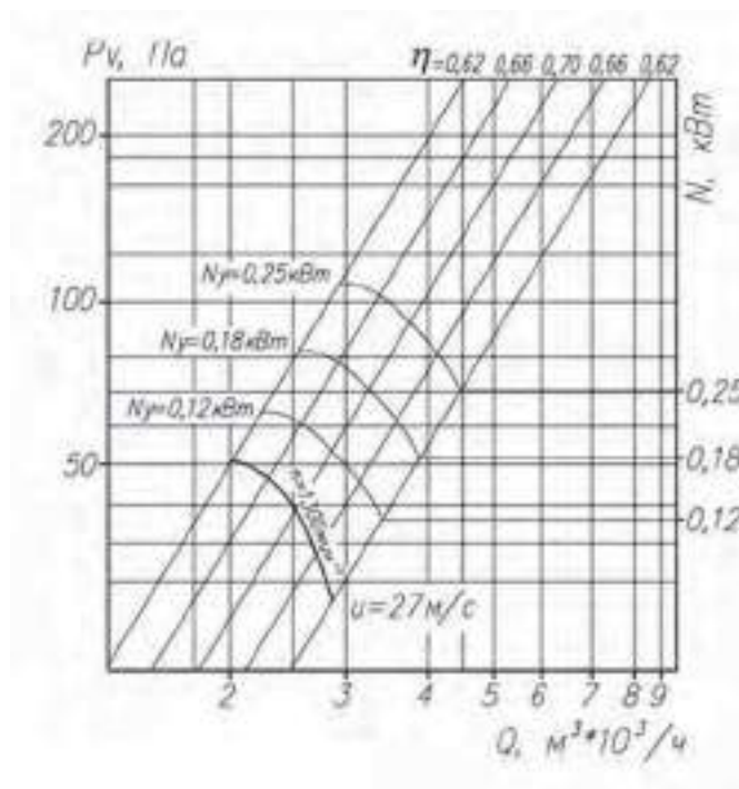
Аэродинамическая характеристика вентилятора ВО 06-300 №3,15
