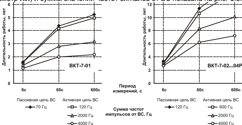
Рис. 1.1 – Зависимость ресурса батареи BKT-7
