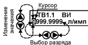
Рис. 3.2 – Пример изменения значения параметра ВИ
