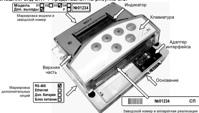
Рис. 2.1 – Внешний вид BKT-7
