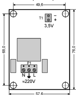
Рис. Н.1 – Внешний вид блока сетевого питания Технические
