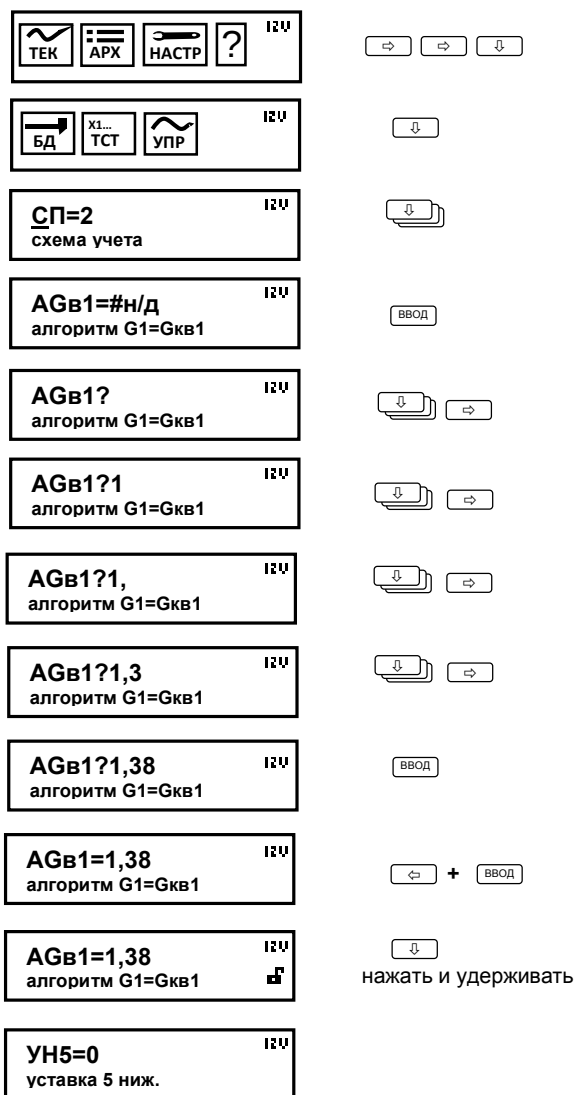
Рисунок 5.6 – Работа с настройками параметрами.
