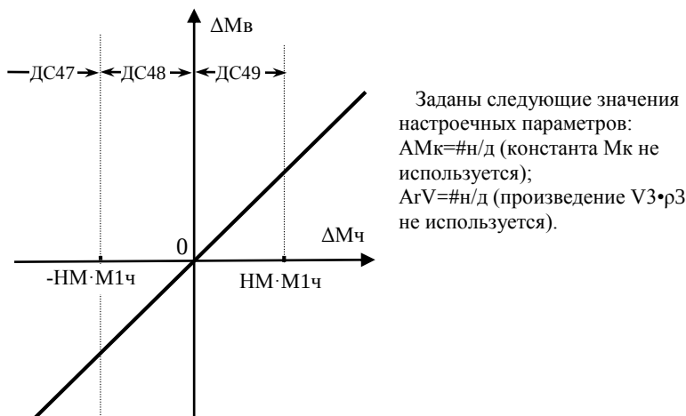
Рисунок 7.4 – Контроль разности часовых масс \Delta M_{\text{ч}} = (M1_{\text{ч}} - M2_{\text{ч}})
