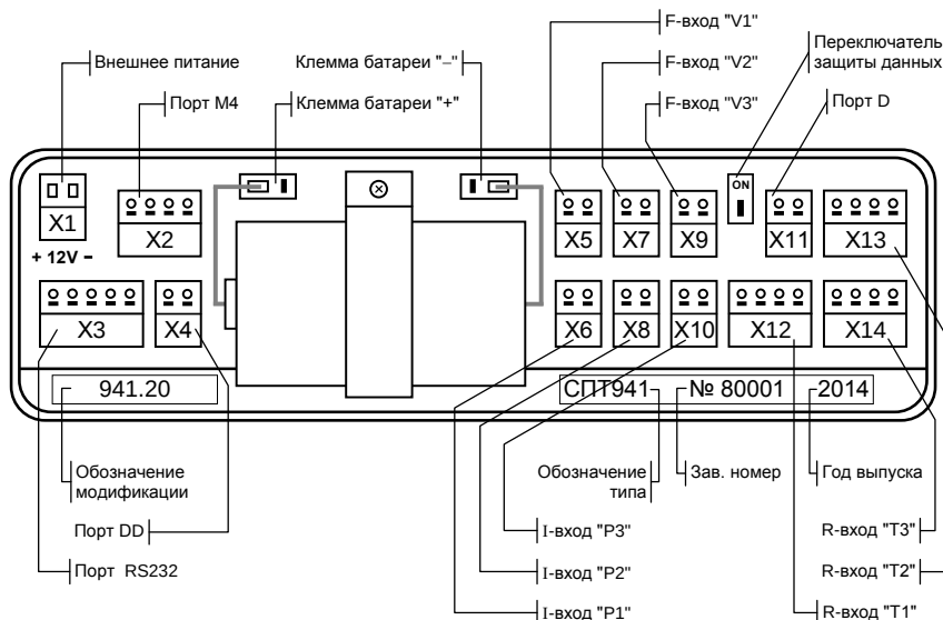
Рисунок 3.3 – Монтажный отсек
