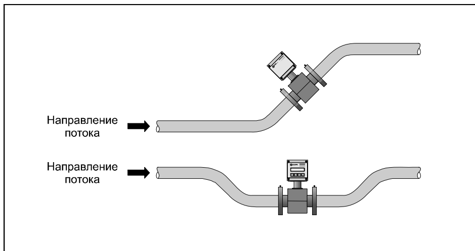
Рисунок 7— Рекомендуемое размещение первичных преобразователей на горизонтальном трубопроводе
