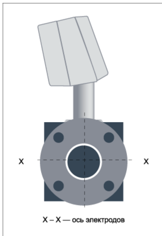
Рисунок 4— Ориентация первичного преобразователя (датчика) расхода относительно продольной оси
