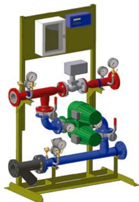
Модуль отопления Зависимая схема со сдвоенным насосом на перемычке
