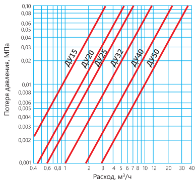
График потери давления многоструйных счетчиков воды
