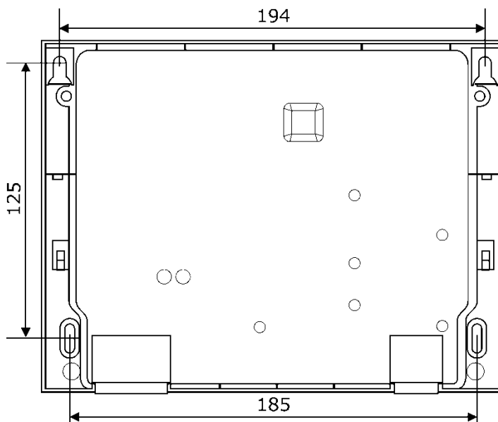
Рис. 4.1 – Схема крепления корпуса ТВ7
