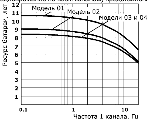
Рис. 1.1 – Ресурс батареи
