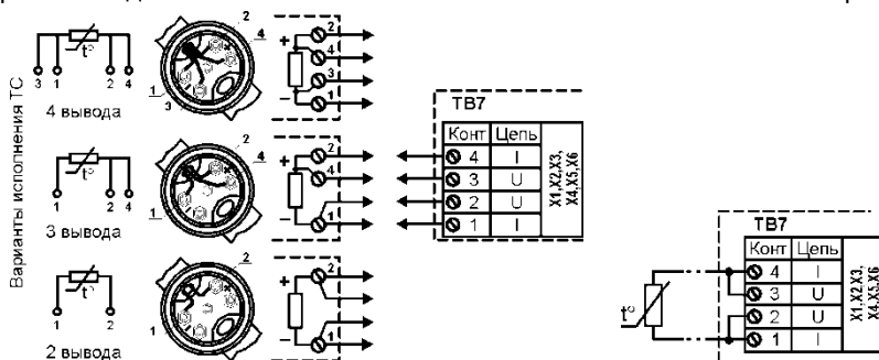
Рис. 4.2 - Варианты подключения ТС
